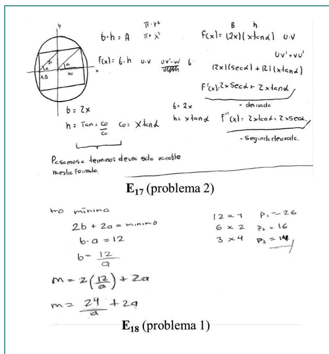
Figura 5. Rutas de solución basadas en procedimientos algebraicos.
